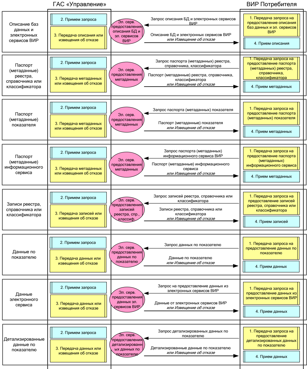
Рис. 2. Схема информационного взаимодействия между ГАС «Управление» и ВИР Потребителей
